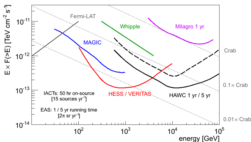
Figura 1: Curvas de sensibilidad en función de la energía y del tiempo de integración para el instrumento LAT del satélite Fermi , los telescopios Cherenkov (Imaging Atmospheric Cherenkov Technique, IACTs) MAGIC, HESS, VERITAS y Whipple, y los detectores HAWC y Milagro (fuera de servicio desde 2008), que detectan la radiación Cherenkov en agua inducida por las partículas de las cascadas iniciadas en la atmósfera por rayos cósmicos o fotones gamma.
