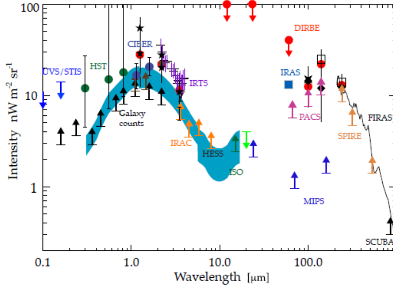
Figura 1: Espectro de la luz del fondo extragaláctico óptico e infrarojo. Figura de Cooray A., Extragalactic background light measurements and applications , Royal Society Open Science, vol. 3, p. 150555 (2016).
